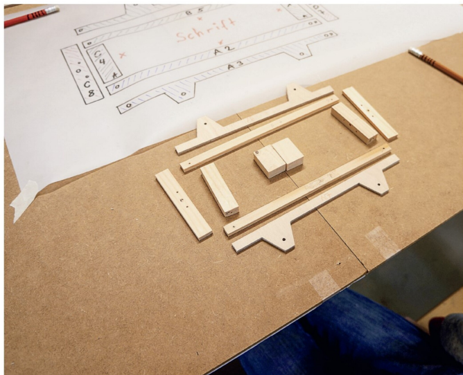
Der Wagenbau wurde Schritt für Schritt, wie hier anhand eines detaillierten Bauplanes, erklärt.
