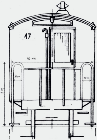
Skizze des modernen Geländers ohne Dachstützen, eingebaut ab 1943.
