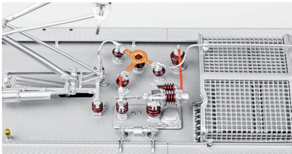
Trennmesser sowie Haupt- und Erdungsschalter funktionieren korrekt.
