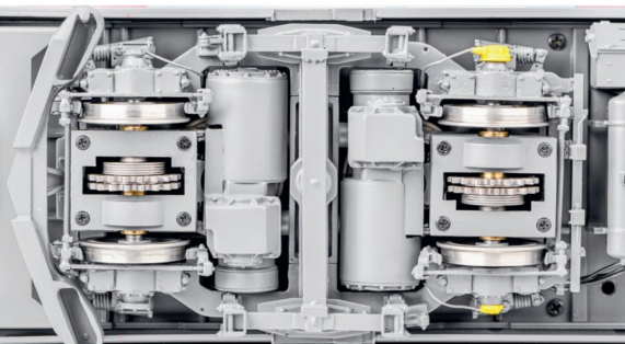
Ein sauber gekapselter Antrieb sorgt für einen ruhigen Lauf.
