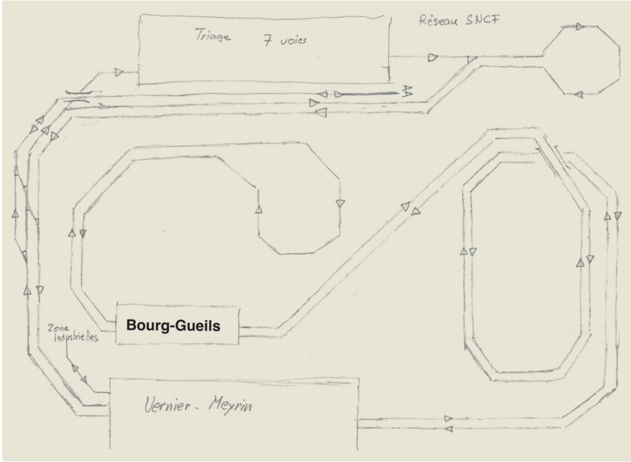
Der Gleisplan des SNCF- Anlagenschenkels.
