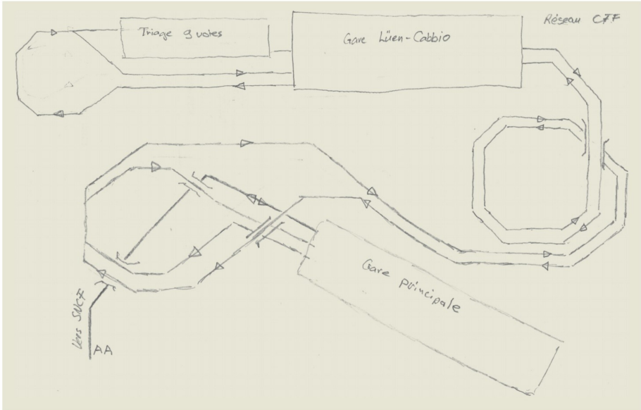
Der Gleisplan des SBB-Anlagen- schenkels.
