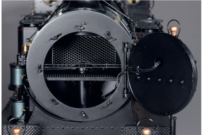
Die Rauchkammerntüre wird durch Drehen der Verschlussriegel geöffnet.
