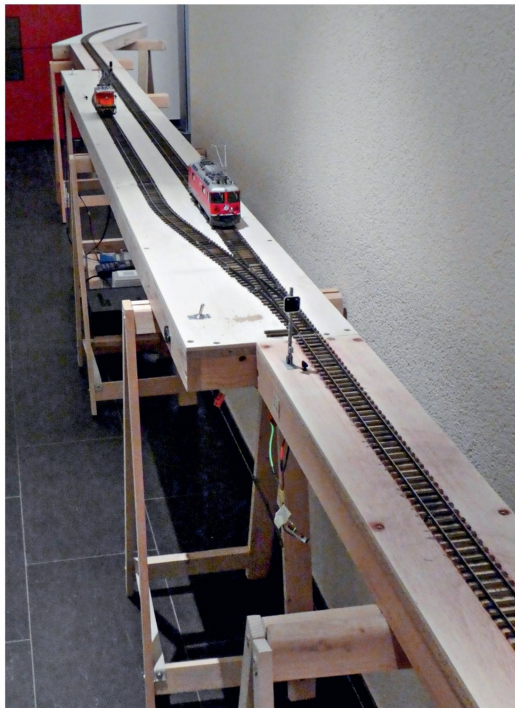
Die Spur-0-Anlage wird auf solchen Holzböckchen aufgebaut.
