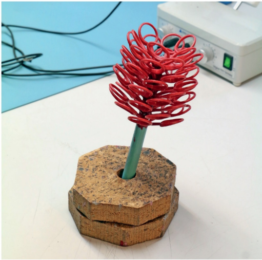
Der fertige Gussbaum, darüber kommt später die Einbettmasse.
