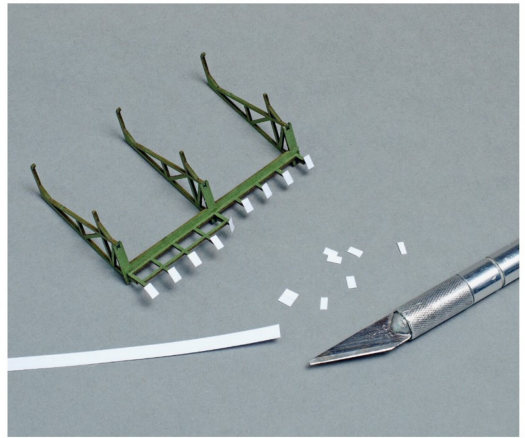
Die Montagebleche entstanden aus kleinen an die Tragekonstruktion angepassten Papierstückchen, die mit Weissleim angeklebt wurden.
