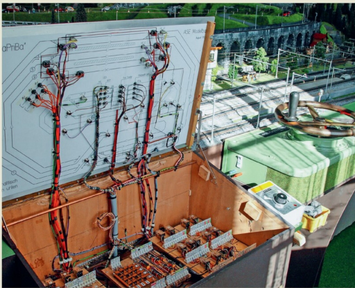
Interessante Einblicke: das ASE-Steuerpult mit Telefonrelais.
