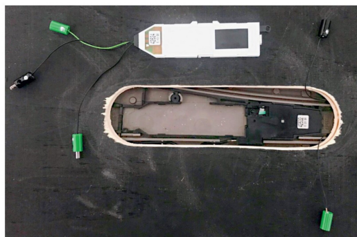
Der noch nicht eingebaute Weichenmotor neben der Öffnung.
