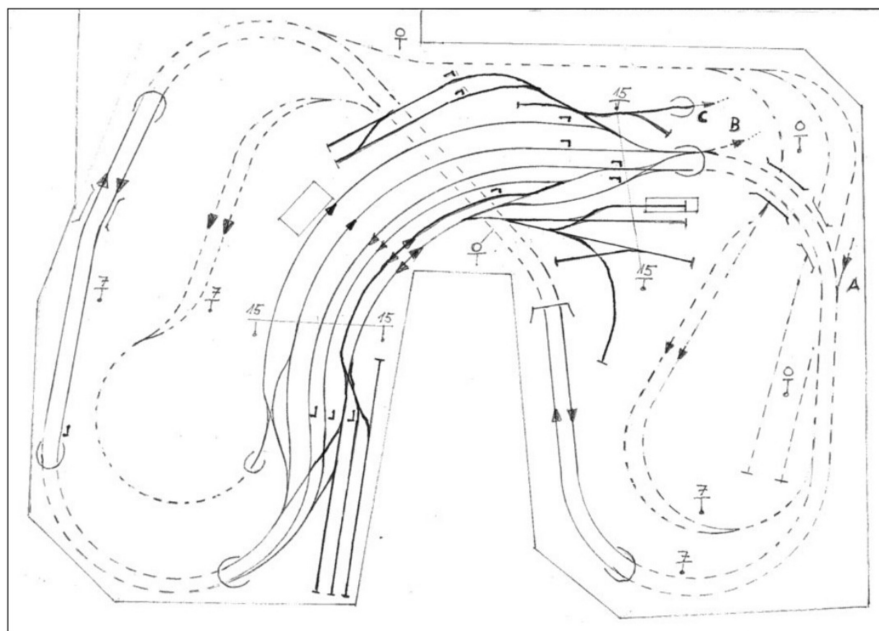
Die zweigleisige Hauptstrecke mit Bahnhof, Depot und Abstellgleisen verläuft in einer gebogenen Acht auf zwei Ebenen übereinander.
