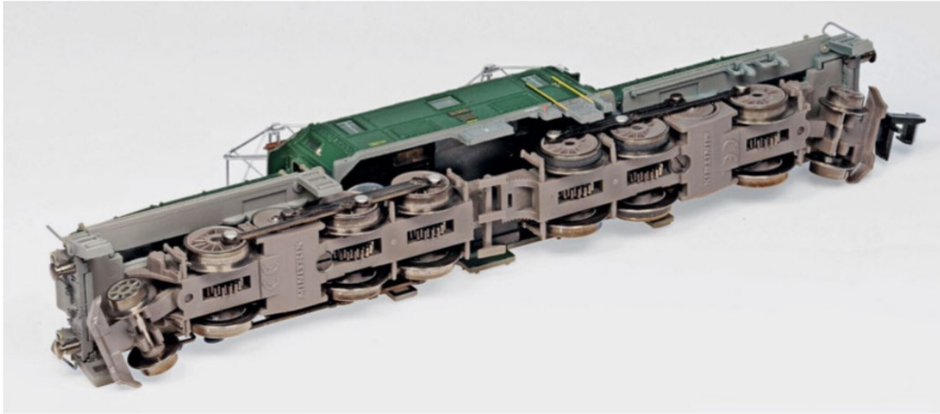
Das N-Modell von unten betrachtet. Alleinstellungsmerkmal des Minitrix-Modells sind die direkt über Metallzahnräder angetriebenen Antriebsachsen.
