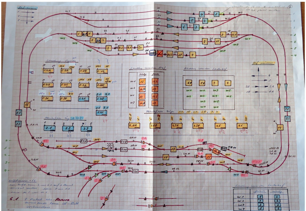
Für jede Ebene hat der Anlagenbesitzer von Hand einen Gleisplan auf Millimeterpapier erstellt und die Schaltungen darin eingezeichnet.
