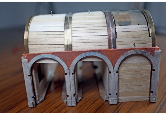
Das erste Projekt der Basler war ein dreiständiger Lokschuppen.
