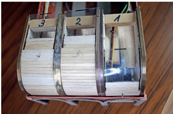
Jedes Tor wird einzeln mit einem Servomotor geöffnet und geschlossen.
