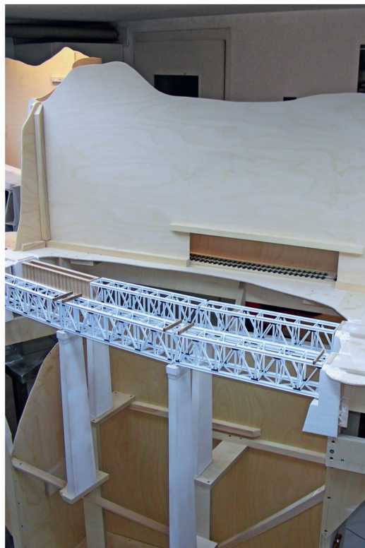
Auf beide Brückenden werden gerade Stahlprofile aufgelegt.
