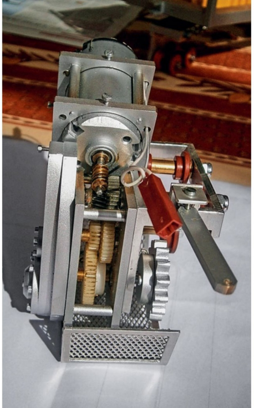
Der Bühler-Motor und die Übertragungsmechanik (Getriebe).
