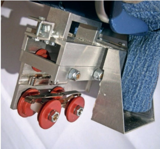
Die Räder der «Lokomotive» mit zwei Stromschleifern für die Stromabnahme.
