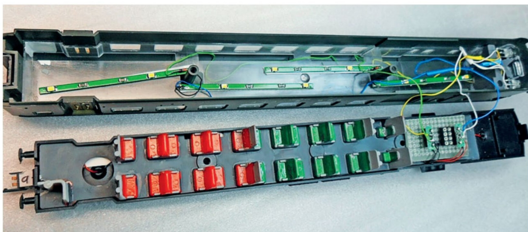
Der fertige Steuerwagen vor dem Zusammenbau. Dass die Innenbeleuchtung mit Reststücken erfolgt ist, sieht man am Schluss nicht mehr.
