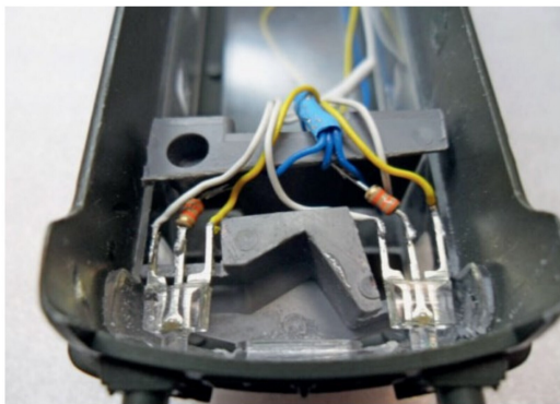
Die LED sind nun fertig verdrahtet und mit Vorwiderständen ausgerüstet.
