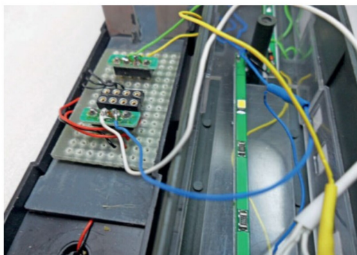
Die Steckergehäuse haben ihren Platz auf der Lochrasterplatte gefunden.
