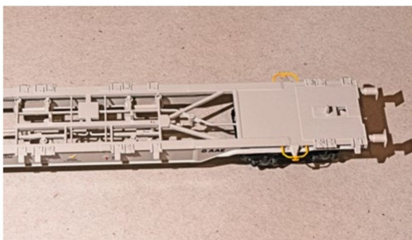
Das Modell zeigt nach Abnahme der Wechselbehälter die gewohnte betriebs-sichere Befestigung ohne den Rahmen für den horizontalen Verlad.
