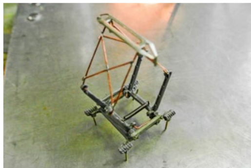
Pantograf in 3-D-Technik erstellt und mit konventionellen Teilen ergänzt.
