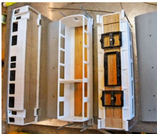
Unter dem Wagenkasten werden Achsaufnahmen angeschraubt.
