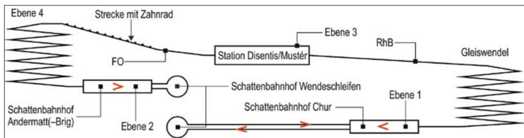
Einen Überblick über die unterschiedlichen Ebenen und Streckenverläufe vermittelt diese schematische Darstellung. Die Wendeschleifen der Schattenbahnhöfe sind unter der Ortsunterführung in zwei Ebenen angeordnet.
