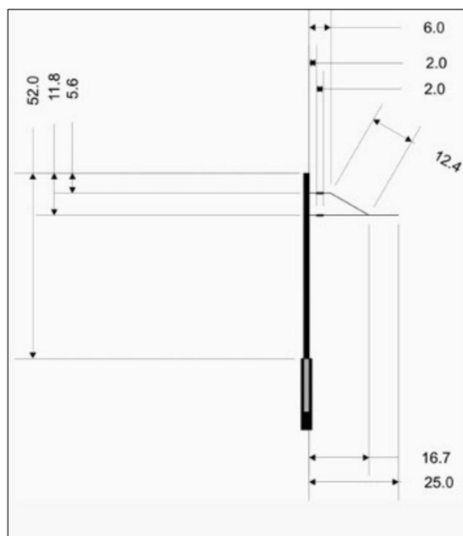
Massskizze des Spezialmastens mit niedrigem Lichtraumprofil.
