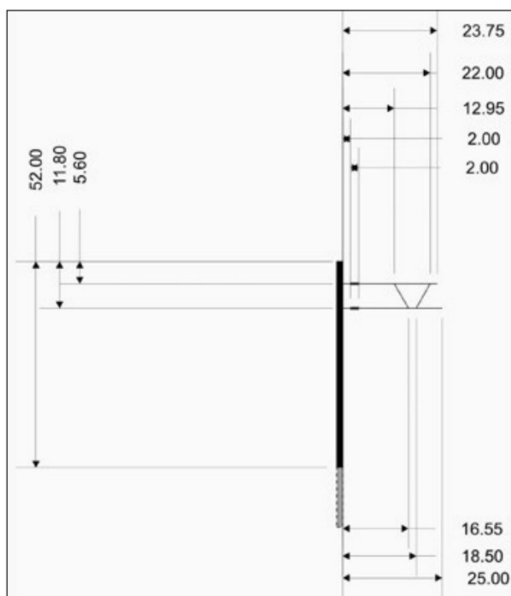
Massskizze des Fahrleitungsmastens in «Normalausführung».
