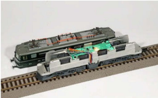
Antiquierte Beleuchtungstechnik mit zwei Birnchen auf der Platine.
