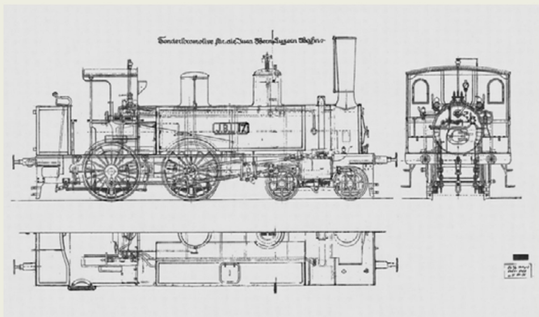
Übersichtszeichnung mit halbem Aufriss und Querschnitt von Lokomotive Nr. 17 der Jura-Bern-Luzernbahn.
