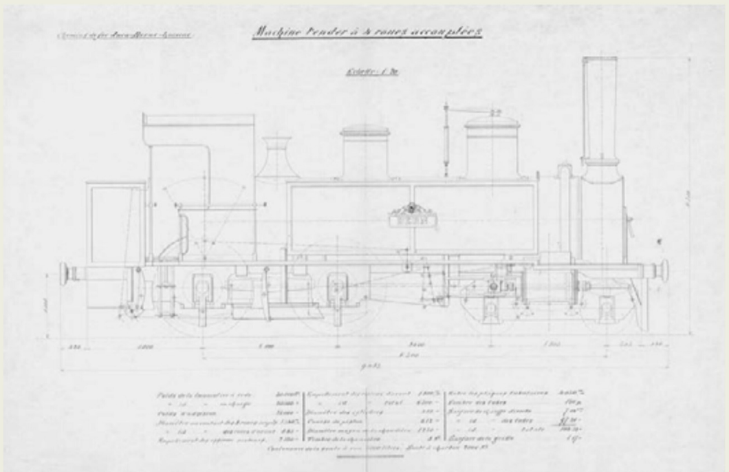
Typenskizze einer Lok der ersten Lieferserie. Die augenfälligen Unterschiede gegenüber dem Werkfoto rühren von nachmaligen Änderungen her.
