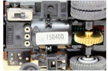
... Getriebe und Antrieb der Hinterachse.
