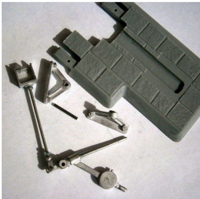
Die Gussteile für einen Weichenstellbock im Massstab 1:22,5.
