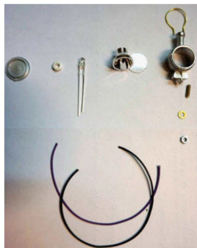
21 Teile, davon zwei aus Weissmetall für eine Loklaterne.
