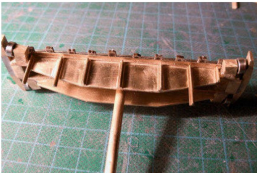
Die beiden Seitenteile entstanden aus Messingblech und -profilen.
