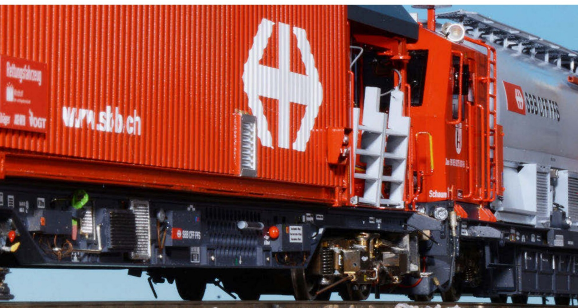
Seitliche Untergestellpartie des Rettungswagens mit aufgeklappten Einstiegen auf die Plattform. Der Rettungswagen kann vom Zug getrennt werden und selbständig
