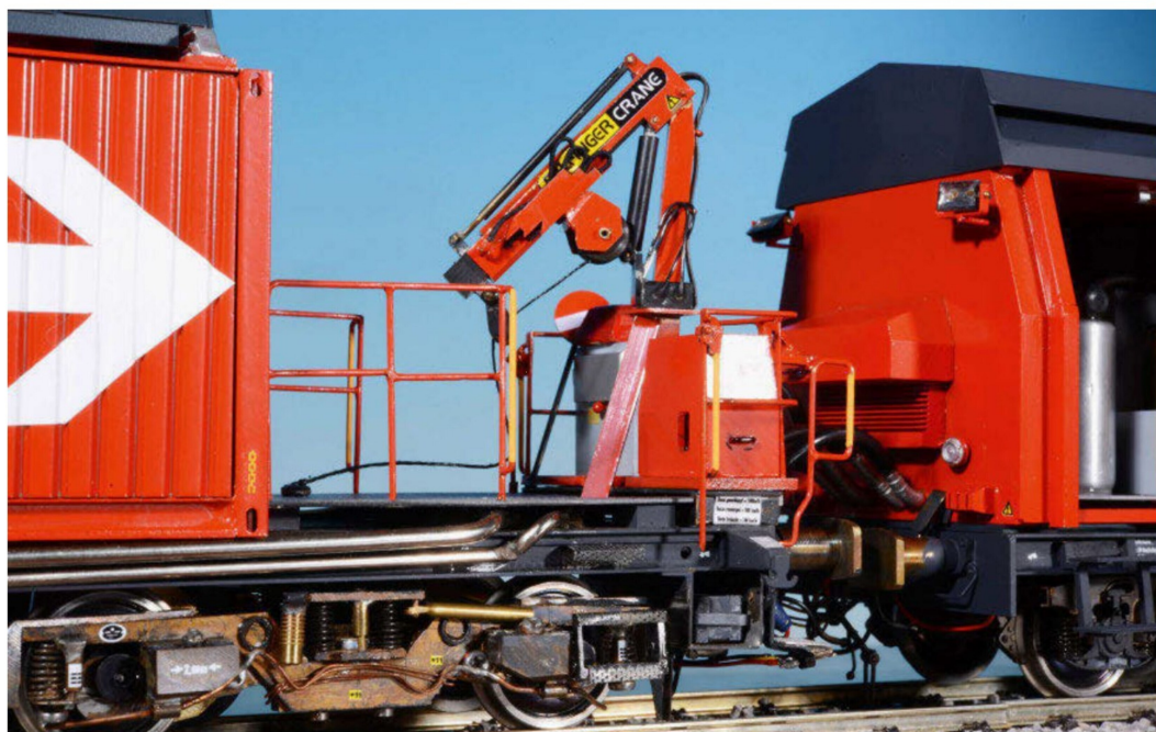
Übergang vom Gerätewagen zum fest gekuppelten Tanklöschwagen mit dem Kran auf der Plattform.
