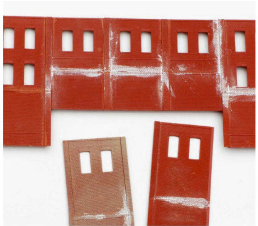
Haupt- und Seitenwände des Industriegebäudes. Kunststoffspachtel wurde an den Trennstellen aufgebracht, damit sich keine sichtbare Spaltbildung ergab.
