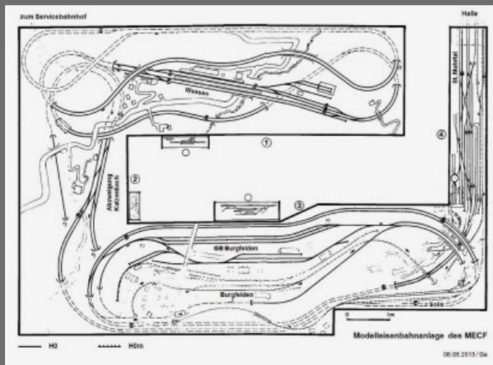
Gleisplan der Anlage. Nicht dargestellt ist die Wendeschleife St. Muhrthal.
