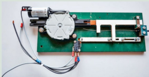
Robuster Weichenantrieb, der unter oder neben den Weichen liegt.
