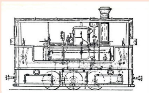
Grobe Planskizze der Berner Kastendampflok. (1)
